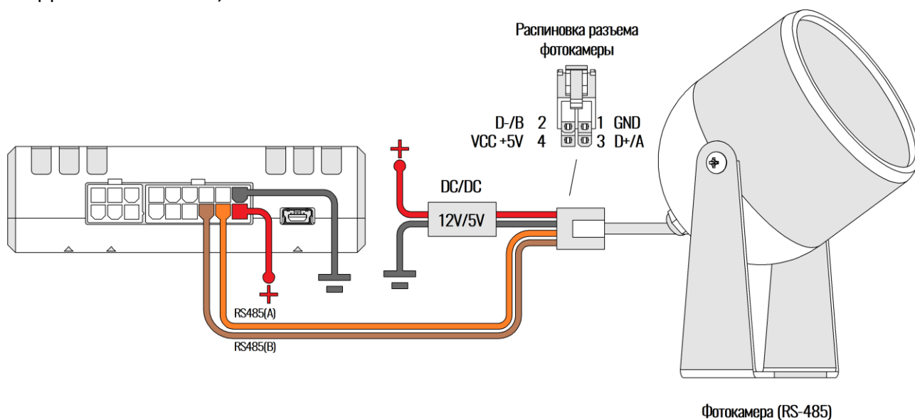
Рисунок 2.30 Подключение фотокамеры JC426F-Q01 с RS-485
