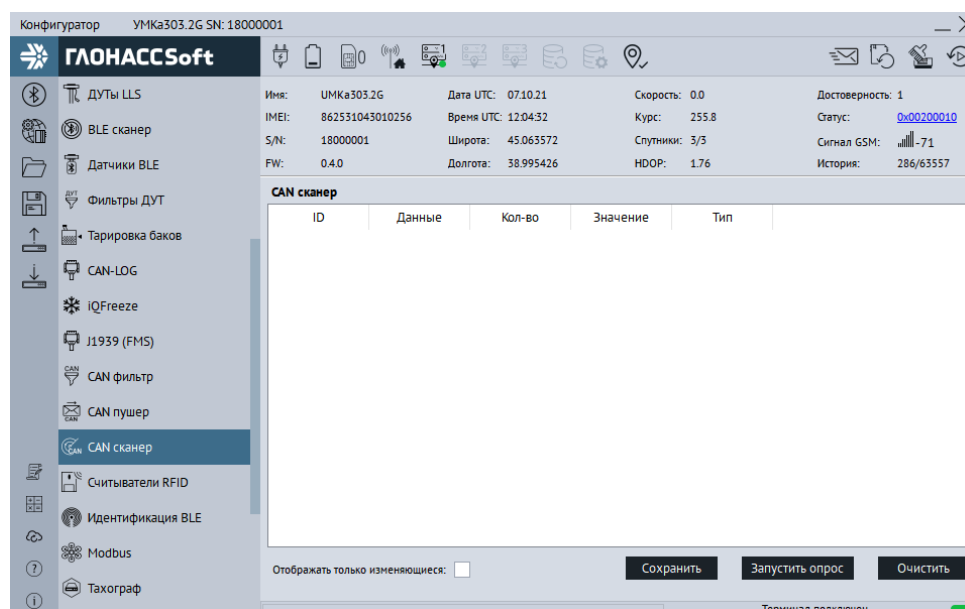
Рисунок 3.36 Вкладка «CAN сканер»
